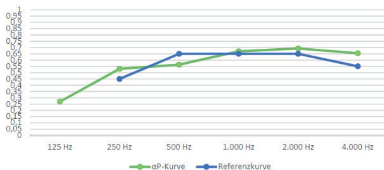
\alpha_P -Kurve
