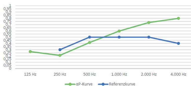
\alpha_P -Kurve
