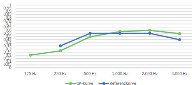
\alpha_P -Kurve
