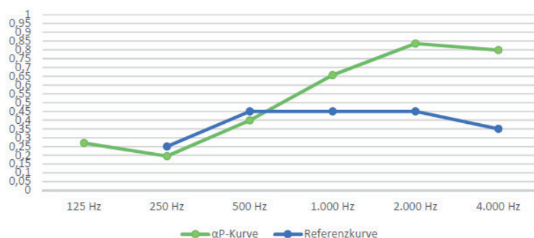
\alpha_P -Kurve
