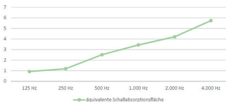
äquivalente Schallabsorptionsfläche (m 2 )
